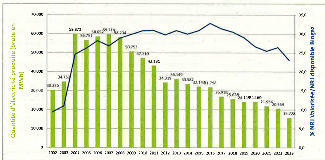
Evolution conjointe de la production électrique annuelle du C.E.Te.M. et du pourcentage d'énergie du biogaz valorisée (courbe bleue) entre 2002 et 2023.
